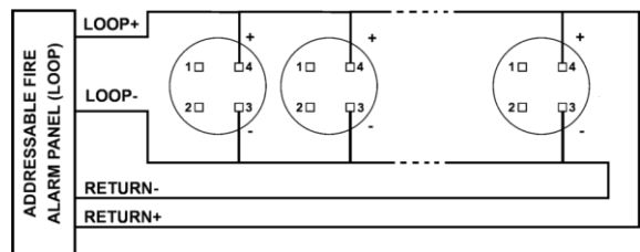
Şekil 1 – Kablolama Bağlantısı
