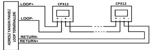
Şekil 1- Kablo Bağlantıları
